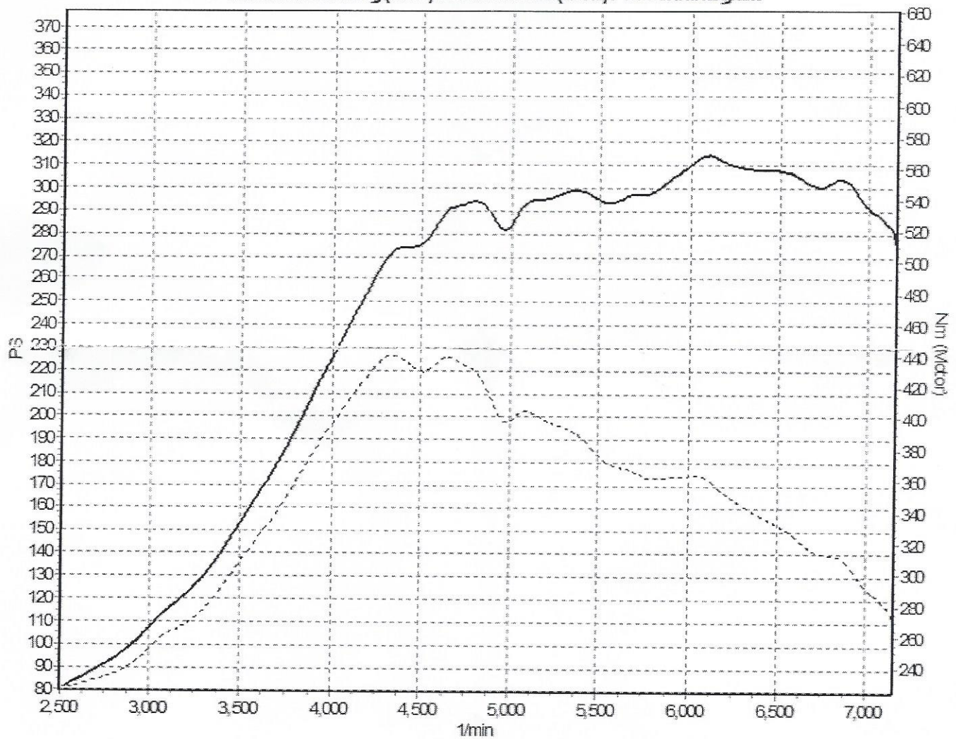
P-max Motorleistung (korr.) / Drehmoment (korr.) / Geschwindigkeit
